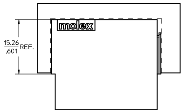
P/N: 46436-9005 SHOWN
