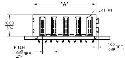
P/N: 46436-9005 SHOWN
