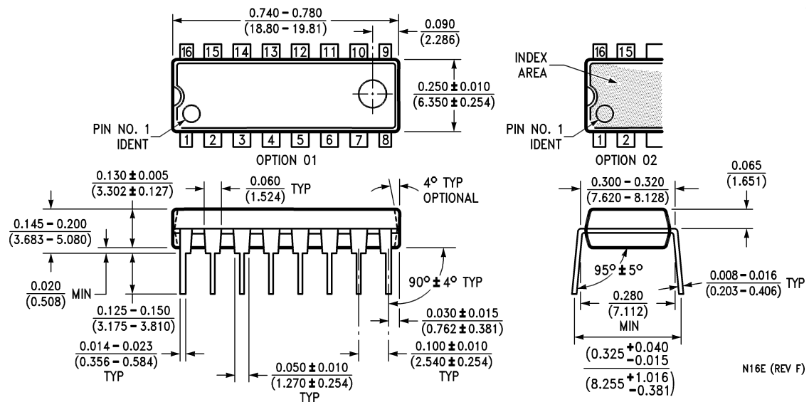
Order Number DS14C232CN NS Package Number N16E
