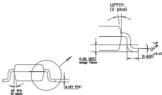
5-Pin TSOT-23 (D5)
