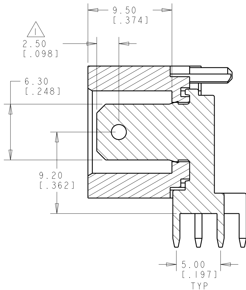
SECTION A-A SCALE 4:1
