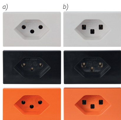
FLF-Steckdosen einmal T13 und T23 Prises FLF une fois T13 et T23 Prese FLF una volta T13 e T23
