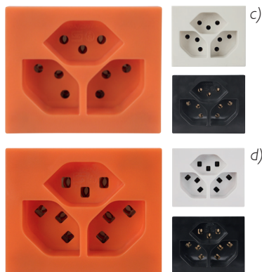
FLF-Steckdosen dreimal T13 und T23 Prises FLF trois fois T13 et T23 Prese FLF tre volte T13 e T23
