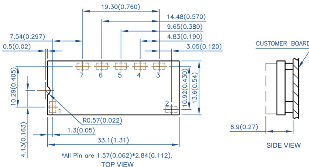
Open Frame Module
