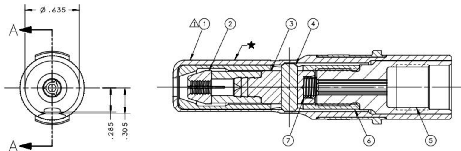
SECTION A-A
