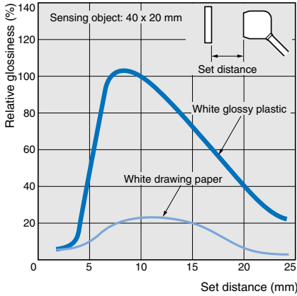
E3X-NL11 with E32-S15L-□
