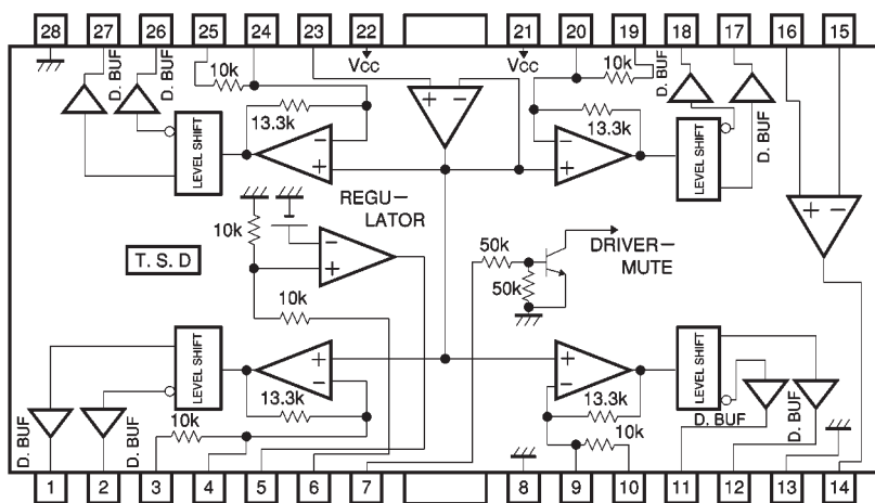
BA6897FP
