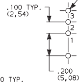
EP11 Models: omit hole 2.
