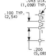
EP11 Models: omit hole 2.
