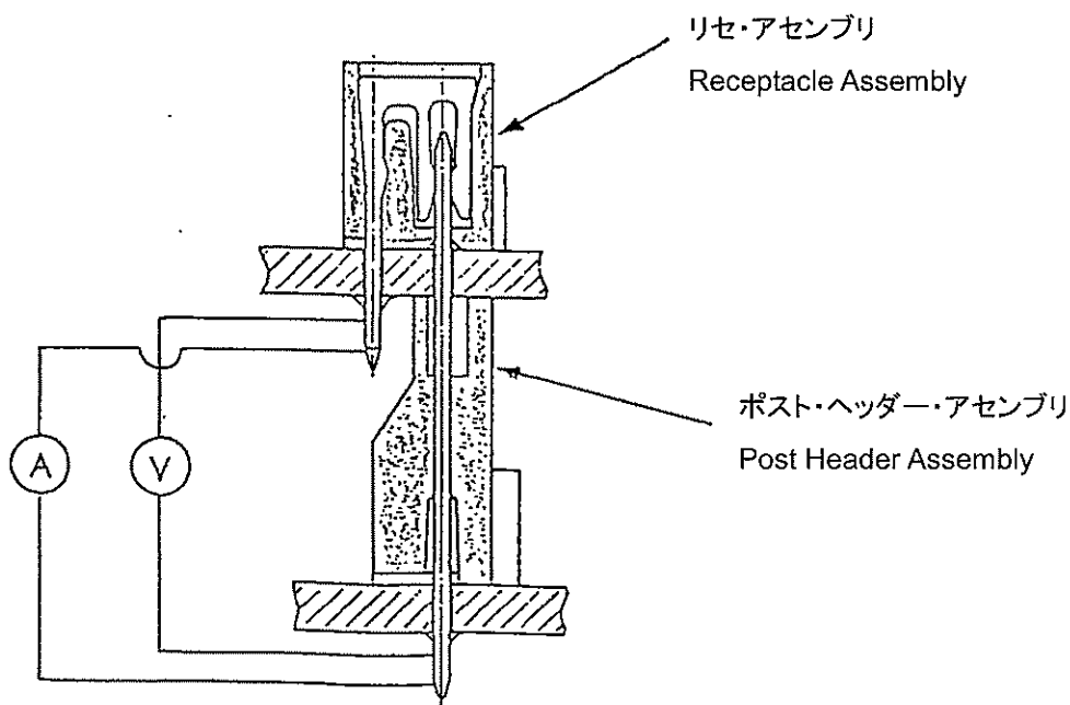
Fig.1 ローレベル総合抵抗測定法
