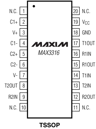
TSSOP
