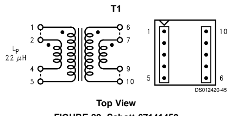
FIGURE 29. Schott 67141450
