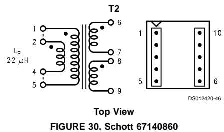
FIGURE 30. Schott 67140860
