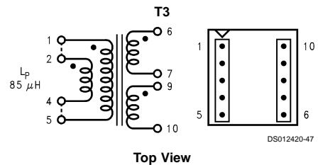
FIGURE 31. Schott 67140920
