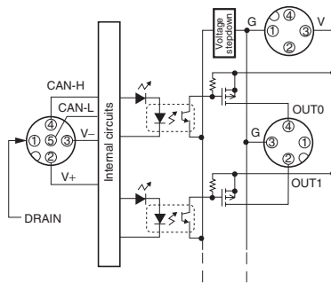
DRT2-MD16CL-1 (PNP)
