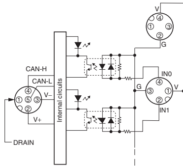
DRT2-WD16CL-1 (PNP)
