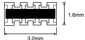
NRSNA6I4 4 Elements
