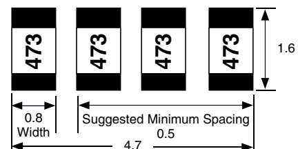
NRC06 (X4) 0603 CHIPS
