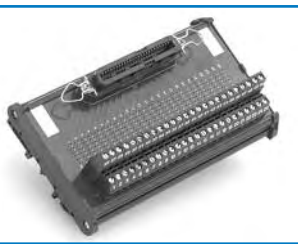
ICN Centronics Module . . . Page 96
