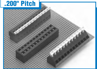
SCM Spring-Clamp . . . . . Page 80 20A / 300V
