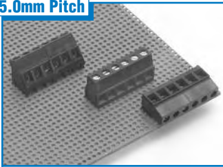
ELM Standard Profiles . . . Page 63 15A / 300V
