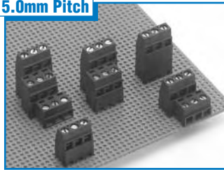
ESLT Multi-tier . . . . . Pages 68-69 13.5A / 300V
