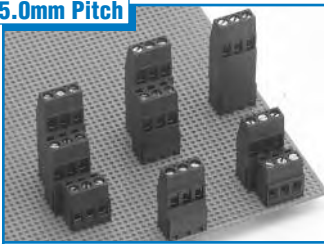
ESTT Multi-tier . . . . . Pages 72-73 24A / 300V
