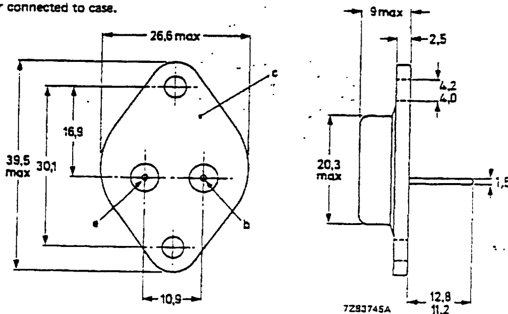
Fig. 1 TO-3.
