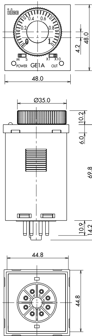
GE1A Timer
