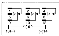
3PDT
