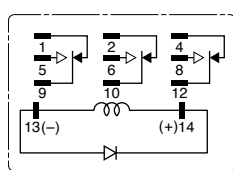
3PDT
