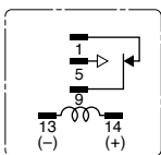
SPDT
