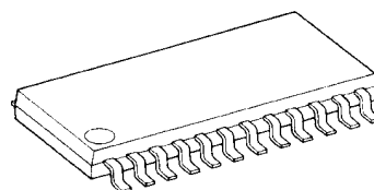
SSOP24-P-300-1.00
