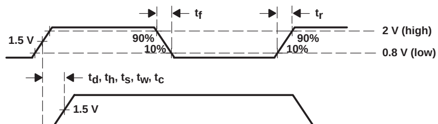
Figure 19. Parameter Measurement
