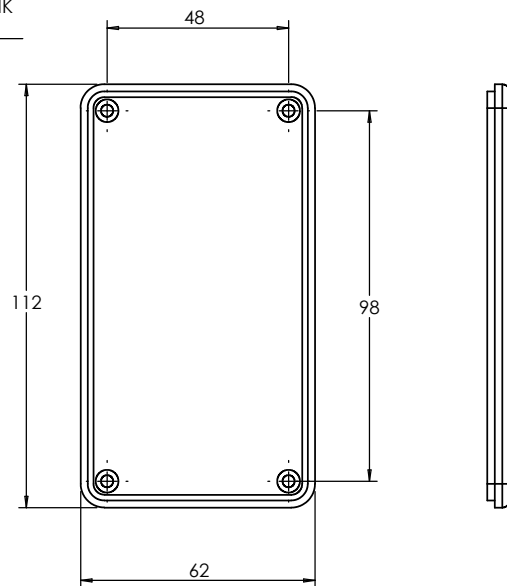
LID
