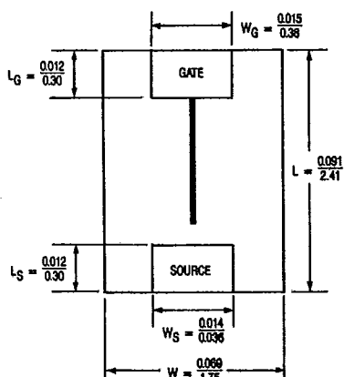
HEX-1: -200V, P-CHANNEL GEN I
