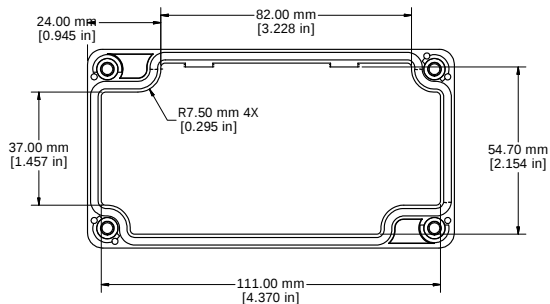
LID - INSIDE
