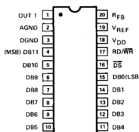
20-PIN HERMETIC DIP (R-Suffix)
