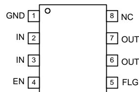
SO-8
