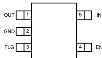
SOT25
