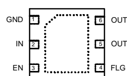
U-DFN2018-6
