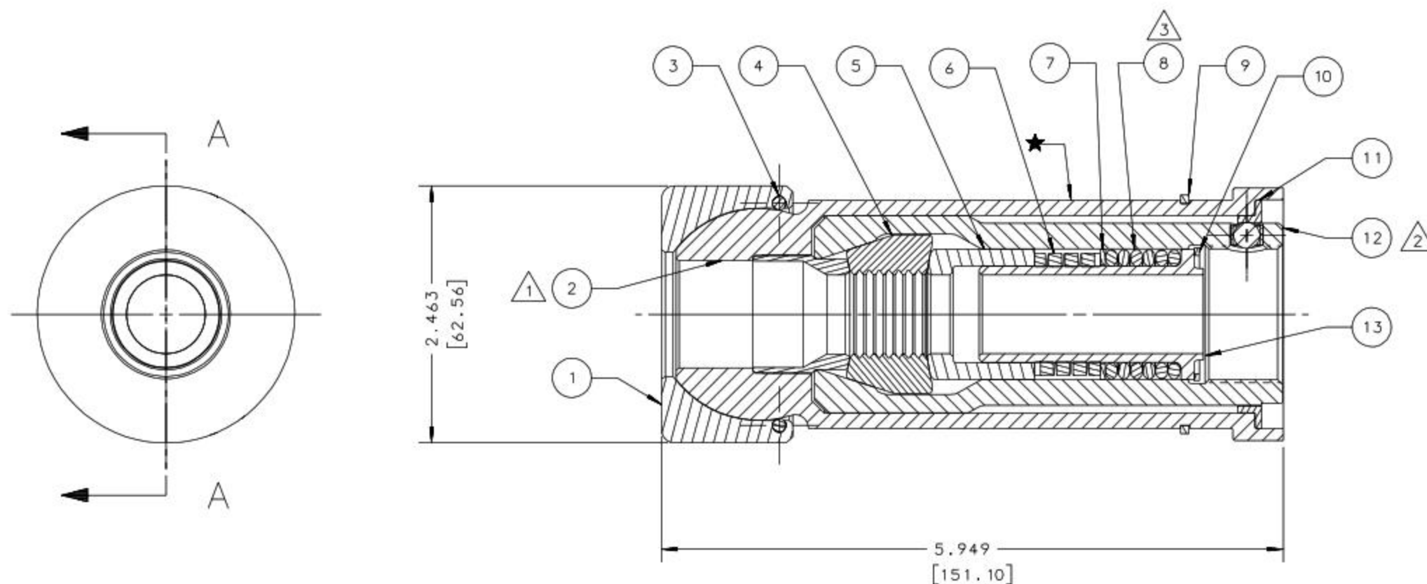
SECTION A-A
