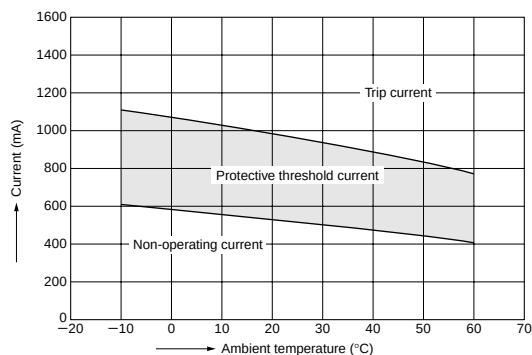
PTGLS5AR0R8M1B53B0
