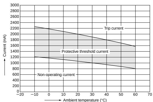
PTGLS8ARR27M1B51B0
