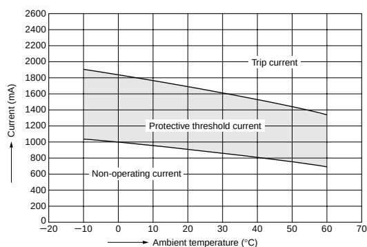
PTGLS7ARR33M1B51B0
