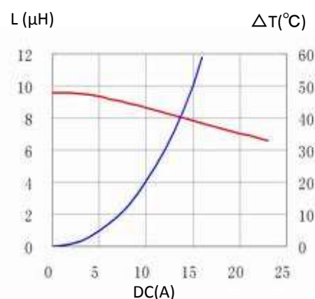
9. 177CDMCCDS-100MC
