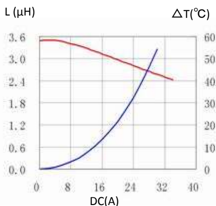
5. 177CDMCCDS-3R3MC
