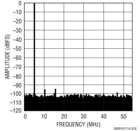
LTM9010-14: 8k Point FFT, f_{IN} = 5\text{MHz} , -1\text{dBFS} , 105\text{Mpsps}
