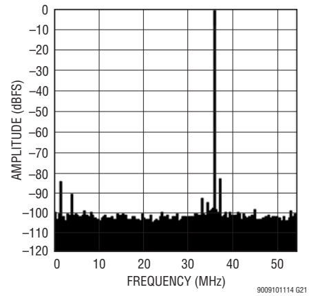
LTM9010-14: 8k Point FFT, f_{IN} = 140\text{MHz} , -1\text{dBFS} , 105\text{Mpsps}
