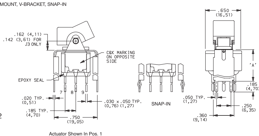
7301J1__BE2 3PDT
