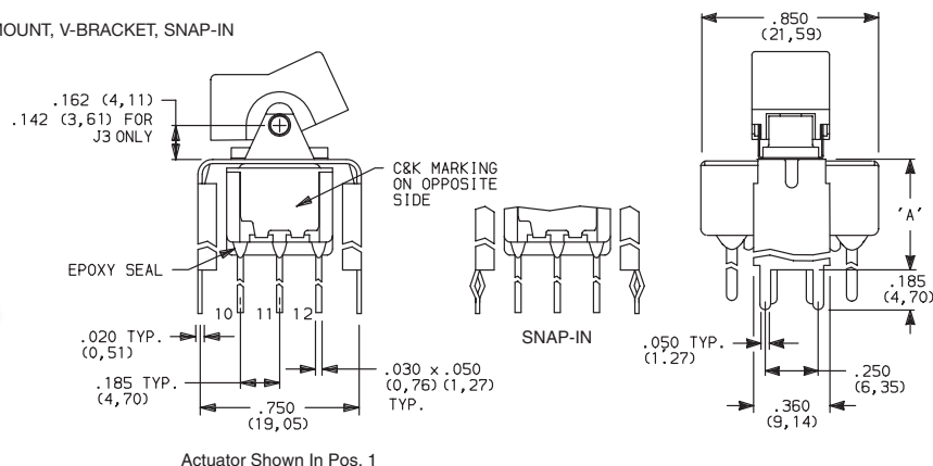
7401J1__BE2 4PDT
