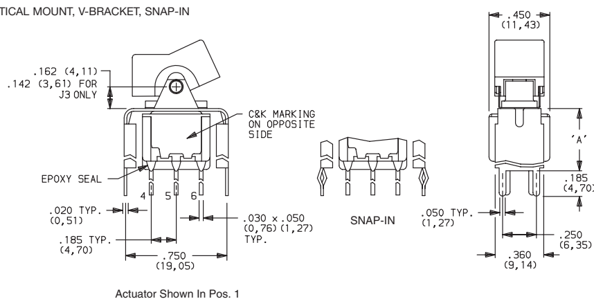
7201J1__BE2 DPDT
