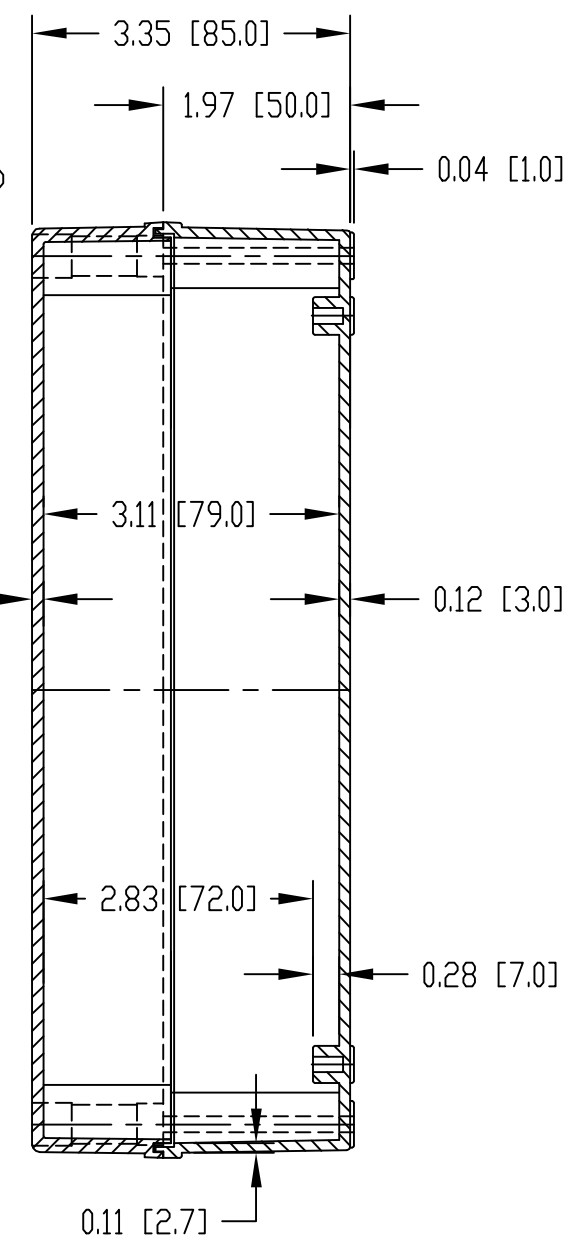
SECTION A-A
