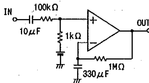
図-26 測定回路図
