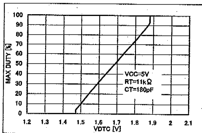
図-16 MAXDUTY-DTC 電圧(設定例)
