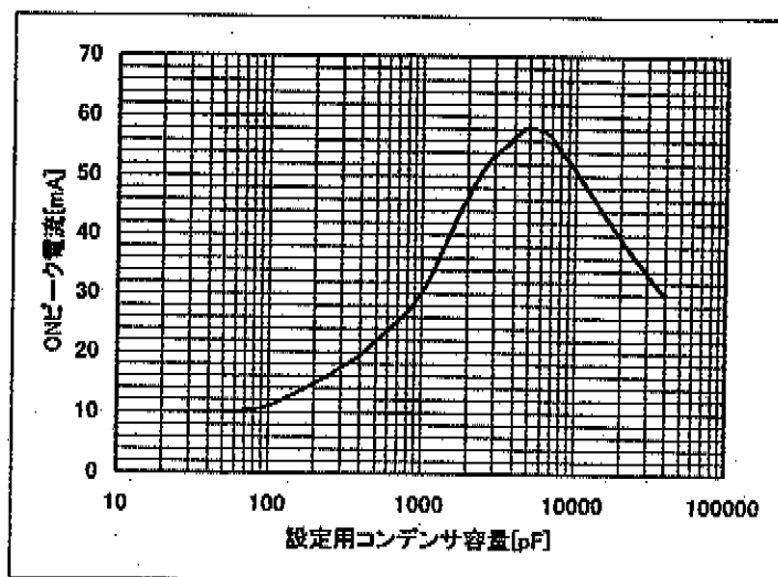
図-19 ON ヒート電流-設定用コンデンサ容量(設定例)
