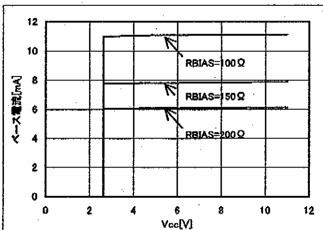
図-27 I_{A-AMP} 電流設定値-電源電圧 (CH2, 昇圧)
