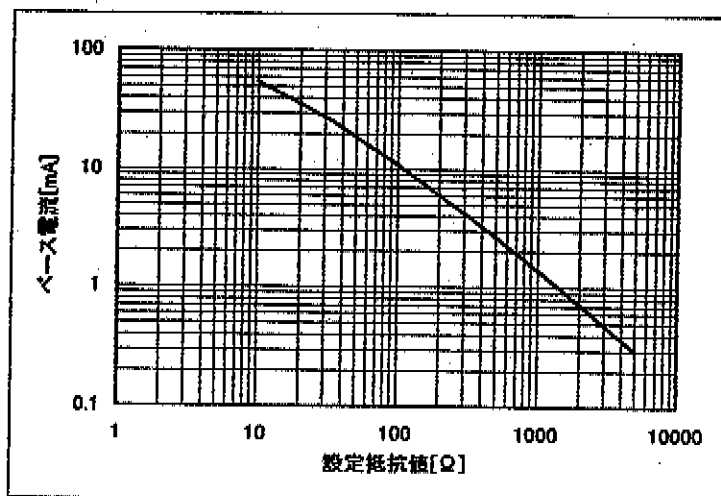
図-18 ベース電流-設定用抵抗値(設定例)
