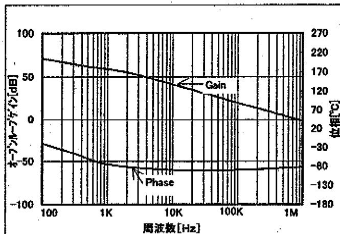
図-25 I_{A-AMP} 利得/位相-周波数特性
