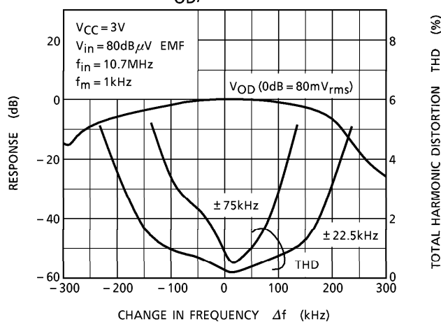
FM (IF)
