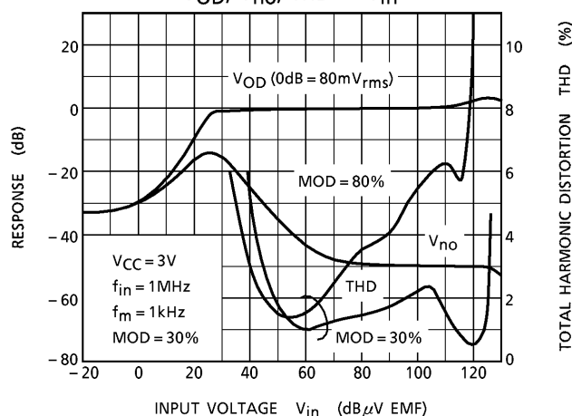
AM
