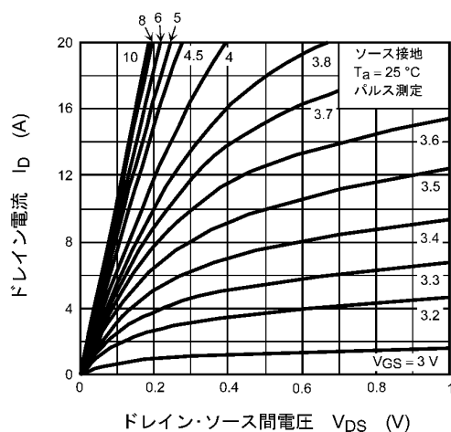
図 8.1 I_D - V_{DS}
