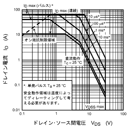
図 8.14 安全動作領域 (最大値 (保証値))
