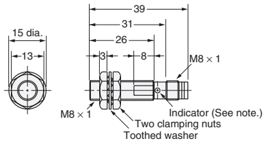
Fig. 28: E2E-X2D□-M3G/E2E-X1R5□-M3/F□-M3
