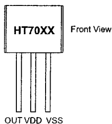
A. TO-92
