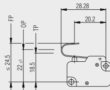
L31: Federhebel
