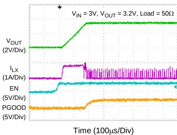
Startup
