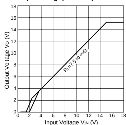
Output Voltage(SI-3152V)
