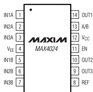
SO/TSSOP
