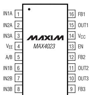
SO/QSOP
