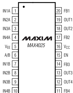
SO/TSSOP
