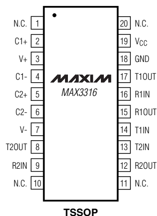
TSSOP
