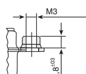
X Clinch nut M3
