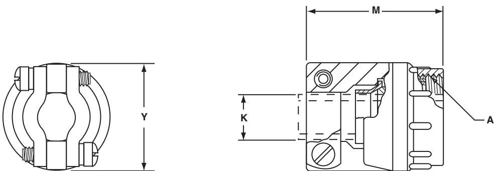
M85049/2-( )C cable clamp
