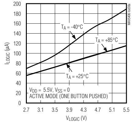
I_{\text{LOGIC}} vs. V_{\text{LOGIC}}
