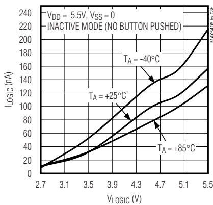
I_{\text{LOGIC}} vs. V_{\text{LOGIC}}
