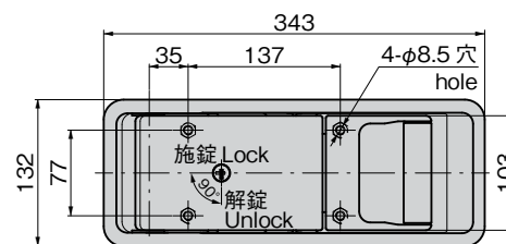
〔FA-877-2〕サイド扉タイプ Side door type
