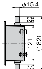
〔FA-877-3-JL〕安全押ボタン付き二重ロックタイプ The double locked-type with safety push button.
