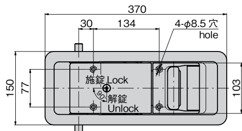
〔FA-877-3-JL〕安全押ボタン付き二重ロックタイプ The double locked-type with safety push button.
