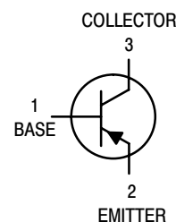
CASE 419-04, STYLE 3 SOT-323/SC-70
