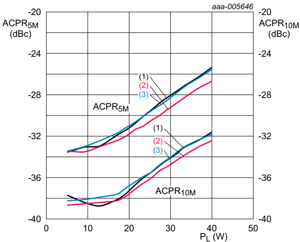
V_{DS} = 28\text{ V}; I_{DQ} = 900\text{ mA}. (1) f = 2500\text{ MHz} (2) f = 2600\text{ MHz} (3) f = 2700\text{ MHz}
