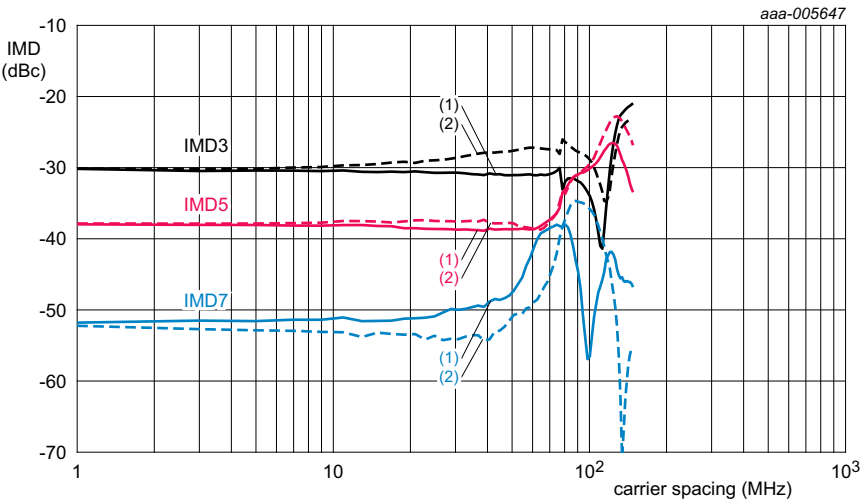
V_{DS} = 28\text{ V}; I_{DQ} = 900\text{ mA}; f_c = 2600\text{ MHz}. (1) IMD low (2) IMD high
