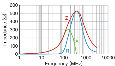
MMZ1608Q221B
