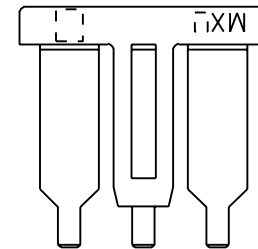
3極品形状 VIEW OF 3 CKT.
